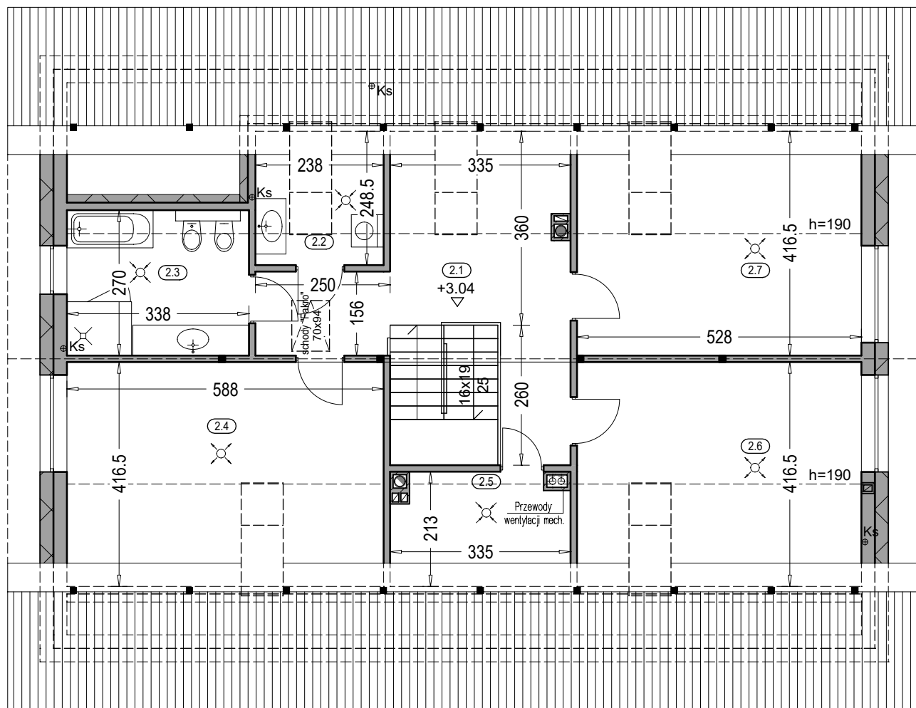
Zestawienie powierzchni strychu
